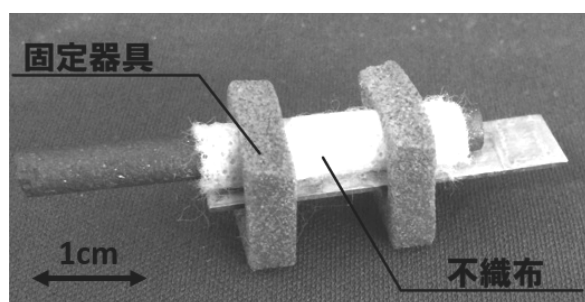
図3 作製した空気亜鉛電池
